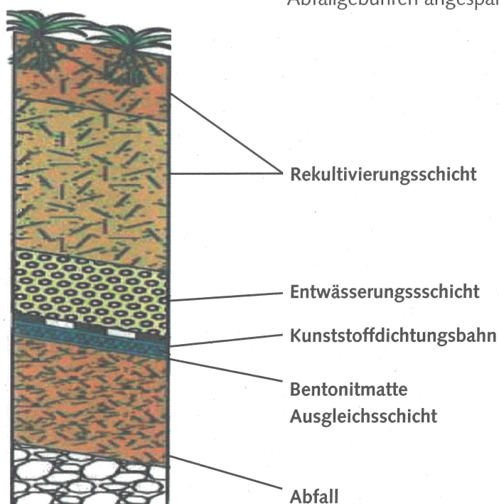
Oberflächenabdichtung
