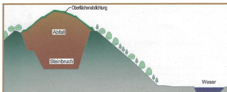
Deponie Querschnitt
